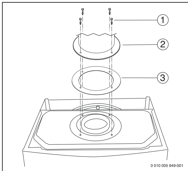
Рис. 14 Крепление переходника
